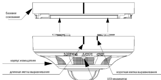
Рисунок 2 – Установка Извещателя на базовое основание.
