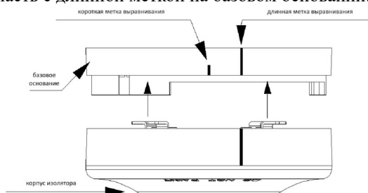
Рисунок 2 – Установка изолятора на базовое основание.
